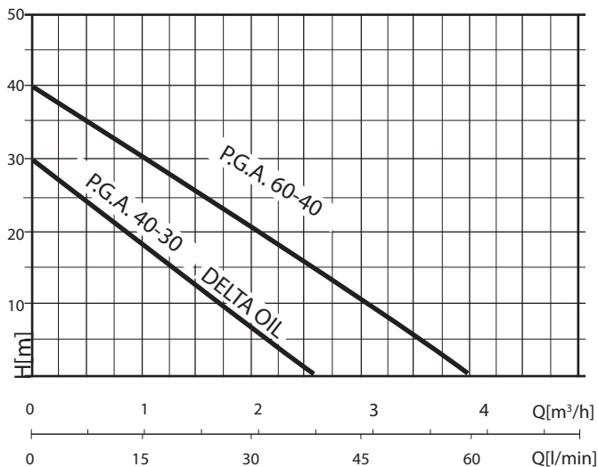
WYKRES PRACY POMPY
